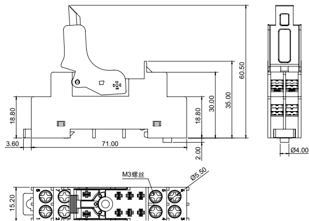
插座外形尺寸图
